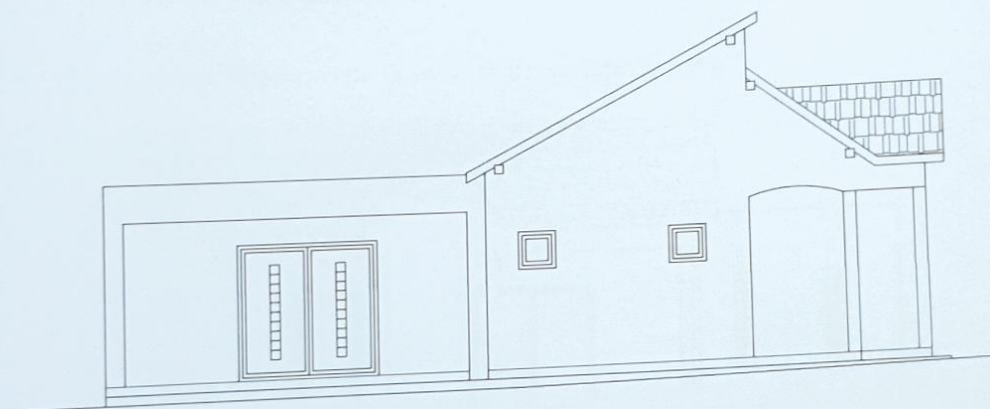
ZAPADNO PROČELJE M 1:100
